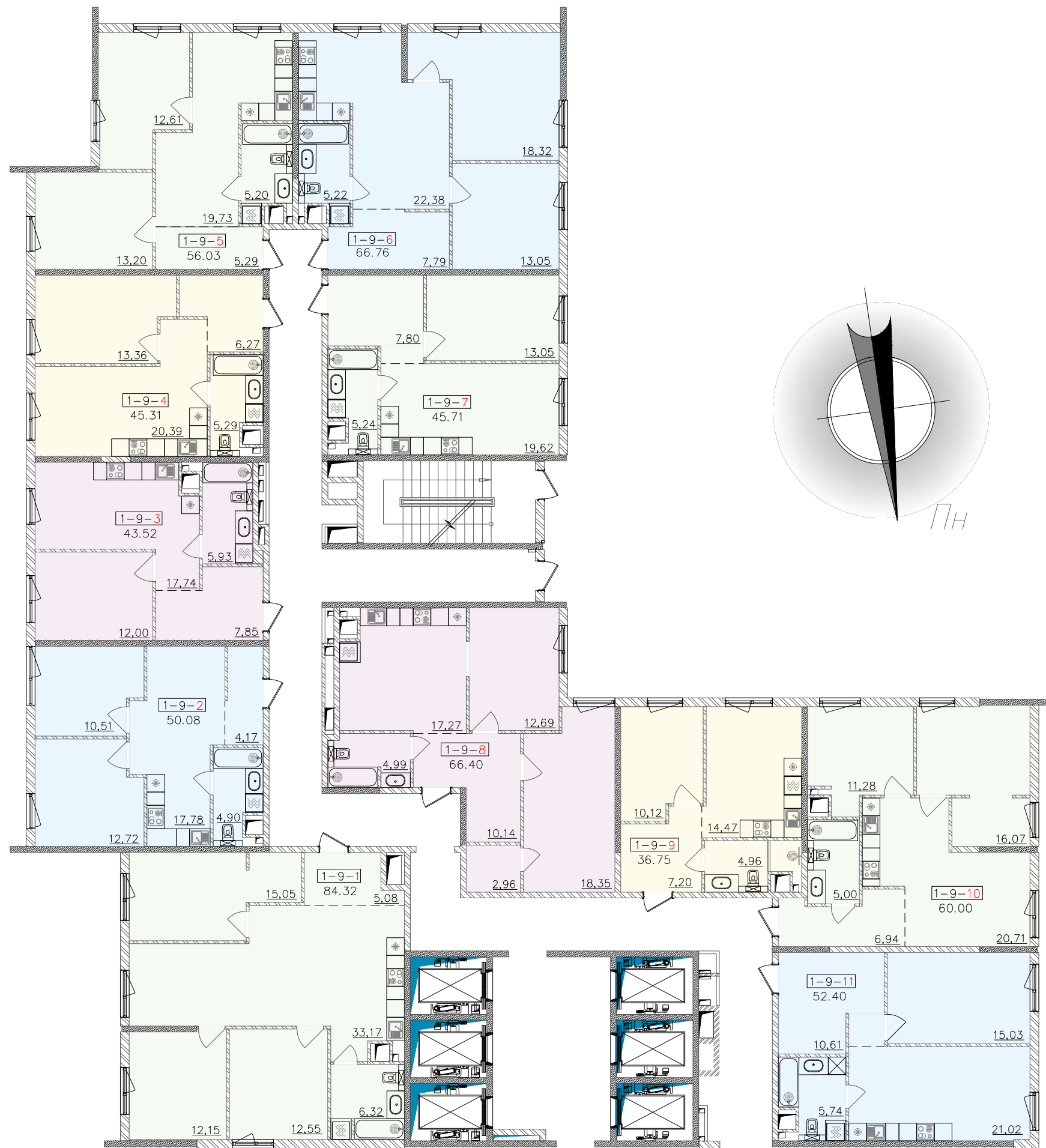
ПЛАН 9 ПОВЕРХУ ЖК "64 Перлина" 1 секція
